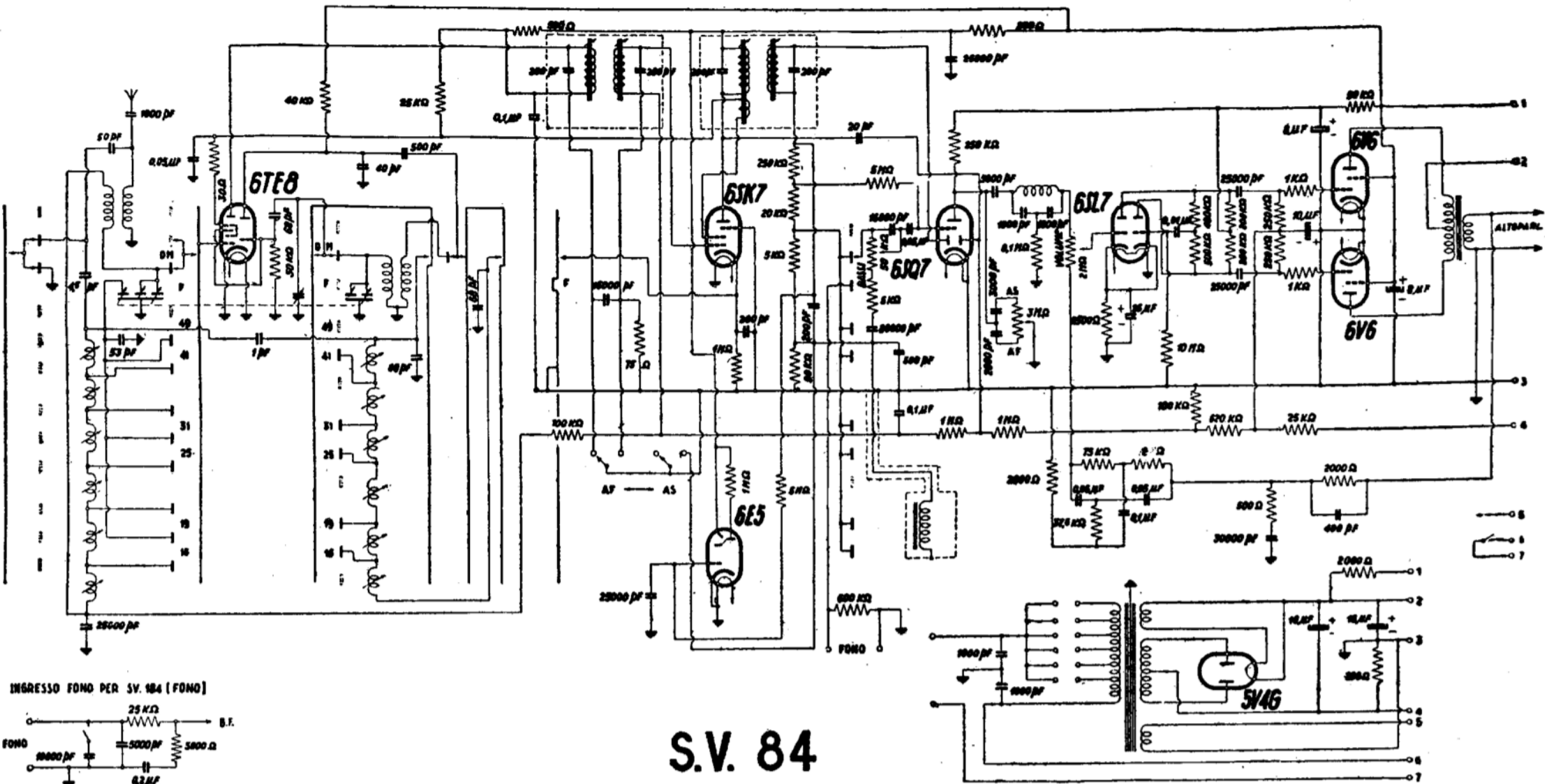
MAGNADYNE RADIO - Modd. SV 84 e SV 184 - Il modello 184 è radiofonografo, v. ingresso nell'angolo sinistro, in basso. Media frequenza 471 kc.
